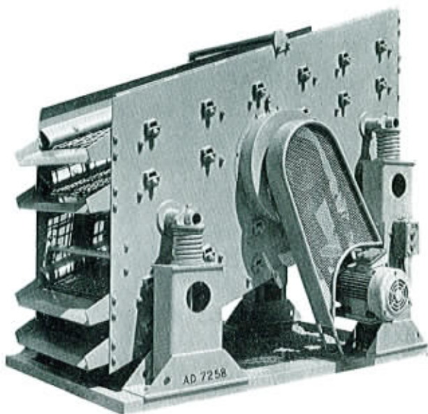
Fig. 5 - Crible V 4 G 75 x 225 sur châssis fixe.
