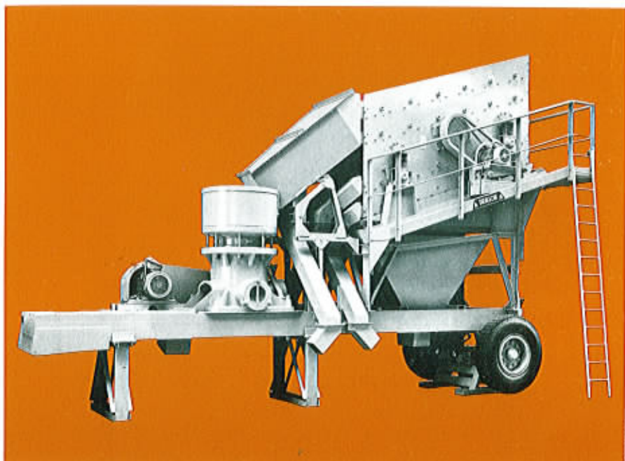
Groupe mobile de criblage-broyage type V100 G3, composé d'un crible DRAGON VP 100 x 300 et d'un gravillonneur giratoire type GS 3.
