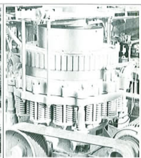
Broyeur GYRADISC 48°
