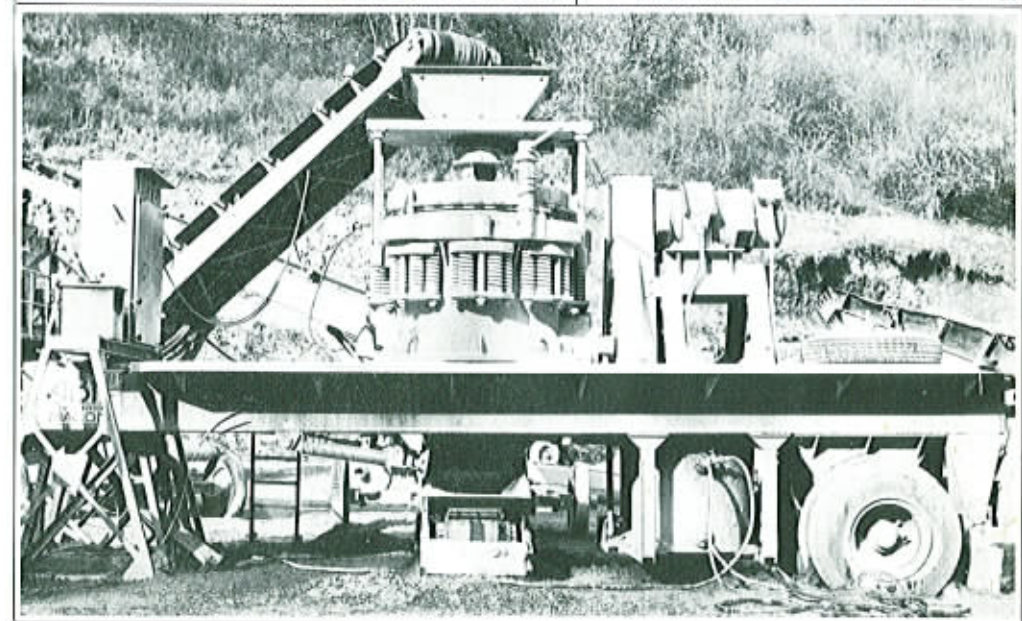
GYRADISC 36° sur groupe mobile
