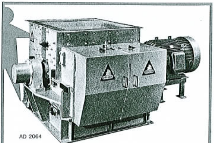
Concasseur spécial à marteaux pour broyage d'ordures ménagères et déchets divers, type ADOM.
