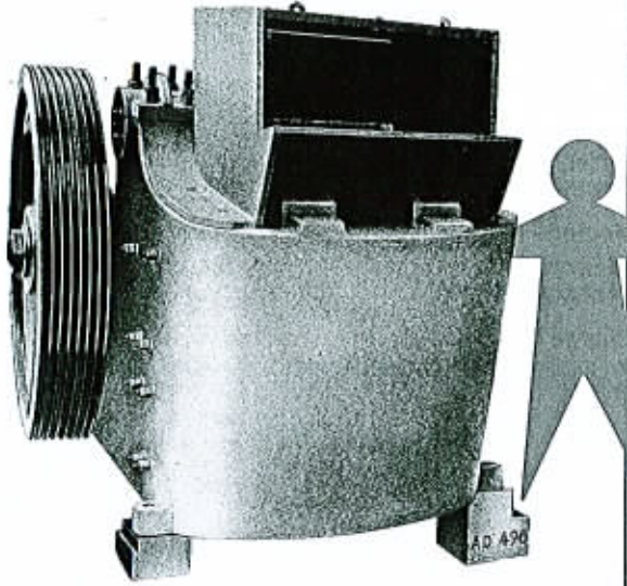
Concasseur spécial super-renforcé type MPR 75 pour traitement de ferro-alliages extra durs.
