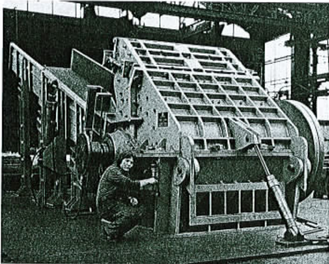
Broyeur à carrosserie type BT.
