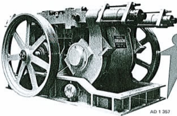
Broyeur à cylindres oscillants type CR 125x65 pour produits durs et abrasifs.
